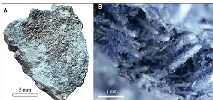
Ротемит – минерал, утвърден от IMA в края на 2024 г., пустиня Негев, комплекс Хатрурим, Израел. Типовият материал се съхранява единствено в НМЗХ – дарение от проф. д-р Ирина Галускина и проф. д-р Евгени Галускин
