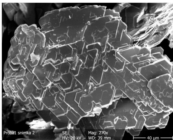
Електронно-микроскопска снимка на осакаит, р-к „Бориева“
