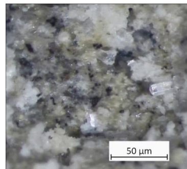
№ 40473 Квадридавин от кариера „Каспар“ (микроснимка)
