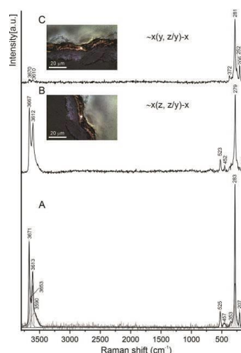
Микрофотография на сканиращ електронен микроскоп и Раманов спектър на точилинит от Яковишкия ултрабазичен масив (изпратени от колегите от Полиа)
