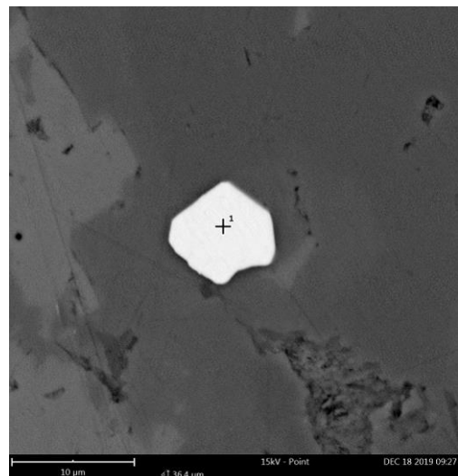
Микрофотографии на сканиращ електронен микроскоп на шпинел и баделеит от находище „Факия“, Бургаско (изпратени от колегите от Полша)
