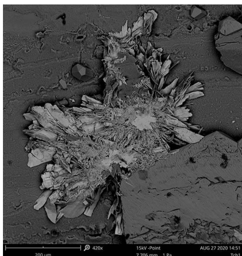
Микрофотография на сканиращ електронен микроскоп и Раманов спектър на точилинит от Яковишкия ултрабазичен масив (изпратени от колегите от Полиа)
