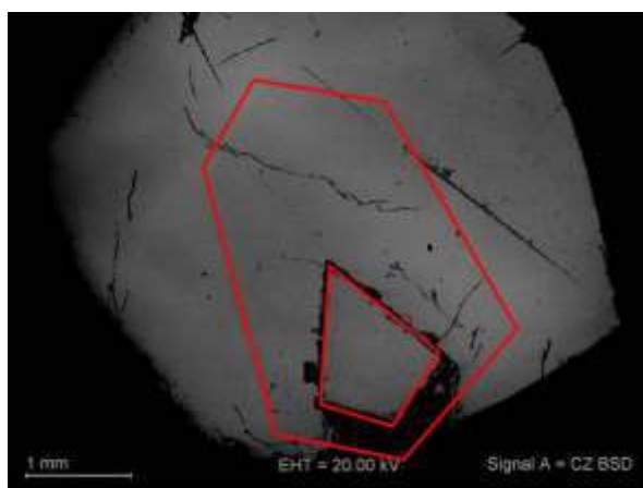
Реконструкция на зоналността
