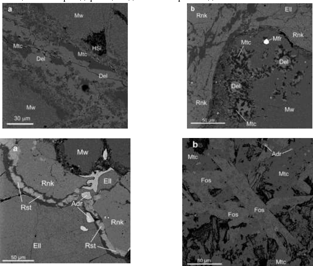
Електронно-микроскопски снимки на новите минерали
