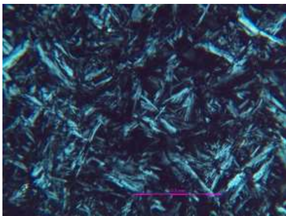
Снимки на поляризационен микроскоп на антигоритов серпентинит (вляво) и на хромитови зърна (вдясно)
