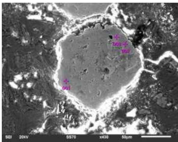
Електронно-микроскопски снимки на хромит (вляво) и на никелови сулфиди (вдясно) с местата на анализите
