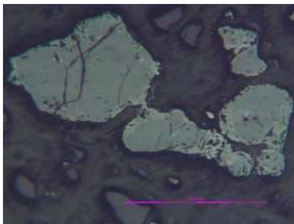
Снимки на поляризационен микроскоп на антигоритов серпентинит (вляво) и на хромитови зърна (вдясно)
